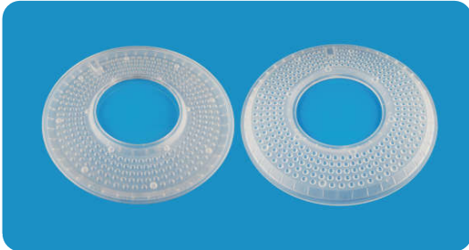
Item No.: HL-ZT60D-K Angle: 60° Dim.: Ø329*H13.1mm Material: PC
