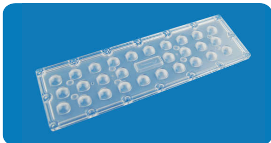
Item No.: HL-260x80-90135D Angle: 90X135° Dim.: L260*W80*H8.3mm Material: PC
